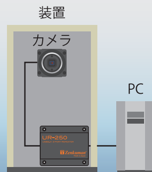
接続例 2
