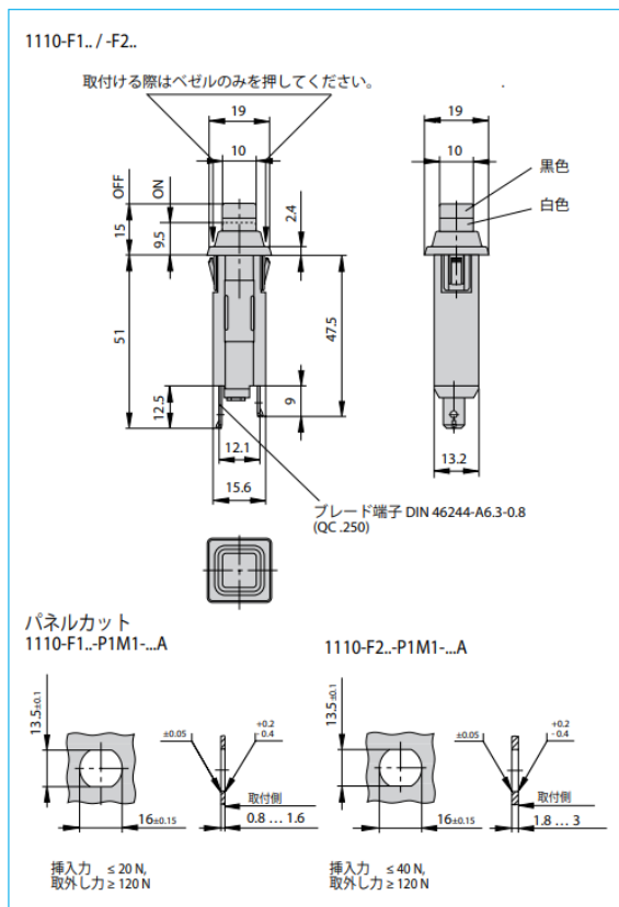
外形寸法図
