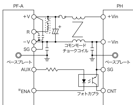
図1-5 PH(280VDC入力)との接続方法
