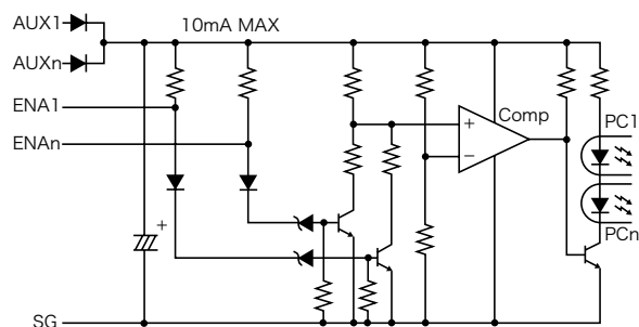
図5-2 N+1並列冗長運転時の信号端子接続
