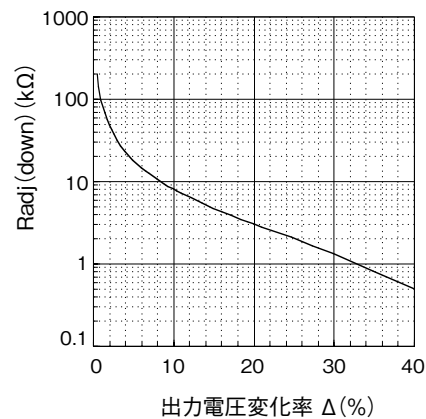
図2-3 Δ (%) 対外付け抵抗(1)
