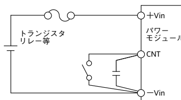
図10-1 CNT接続例(1)
