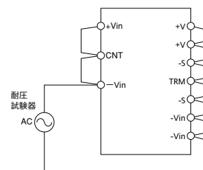
図19-1 入カ-出力間耐電圧試験方法
