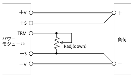
図2-2 可変抵抗接続(1)
