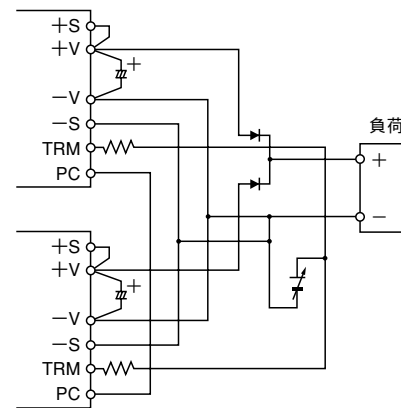
図4-4 外部電圧印加による出力電圧可変が可能な N+1 並列冗長運転
