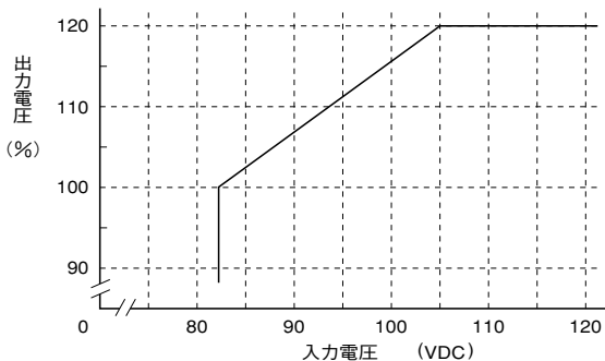
<110VDC入力>
