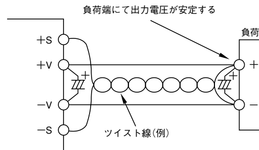
図9-1 リモートセンシングする場合
