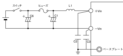
図1-3 スイッチ使用時の入力フィルター
