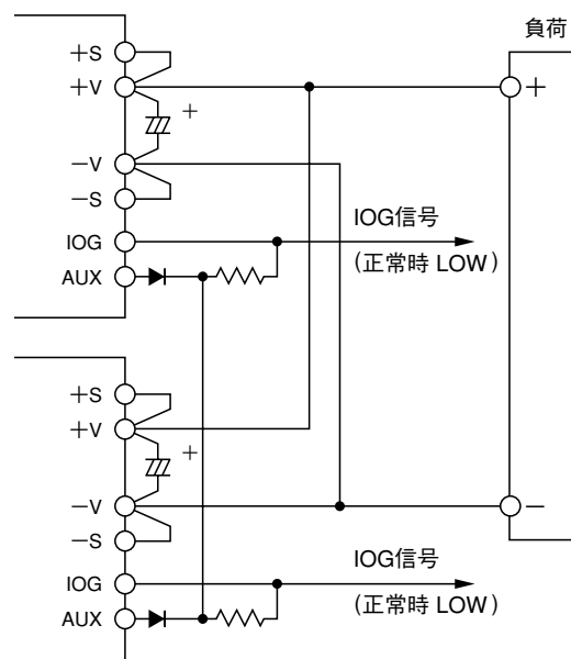
図13-1 IOG端子接続例
