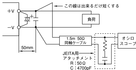
図3-1 最大出力リップル電圧(含ノイズ)測定方法
