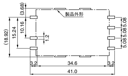
推奨基板取付け寸法
