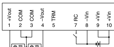
端子接続
