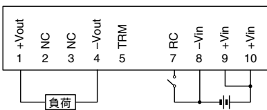
接続図
