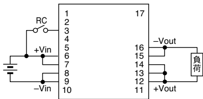
接続図
