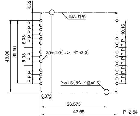
推奨基板取付け寸法
