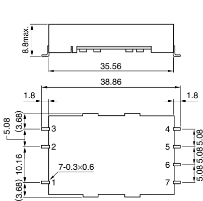
形状・寸法
