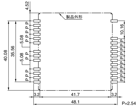
推奨基板取付け寸法
