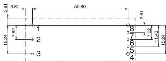
基板穴 (上面視)
