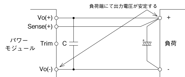
図10-3 リモートセンシングする場合
