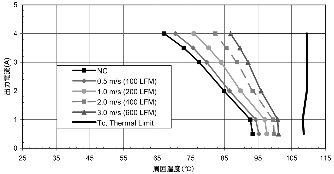
図A-8 iEA4W004A120V-003-R 出力電流ディレーティングカーブ
