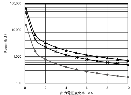
図6-4 △(%)對外付け抵抗
