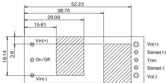
パワーモジュールパターン配線禁止領域(上面透視図)
