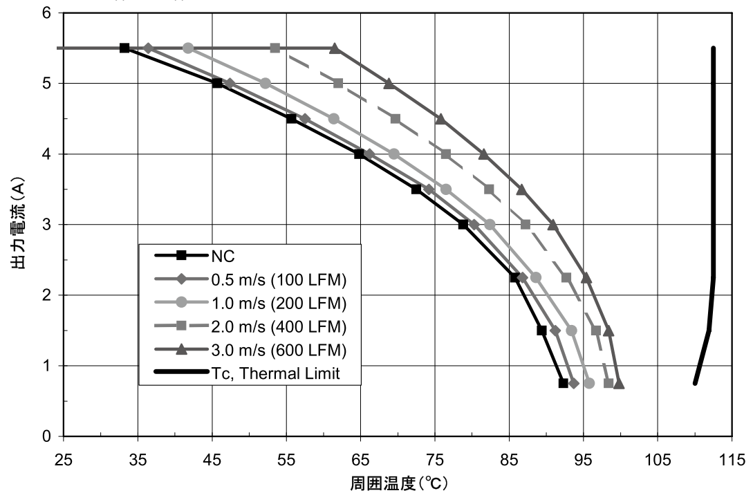
図A-10 iEE48006A120V-003-R 出力電流ディレーティングカーブ
