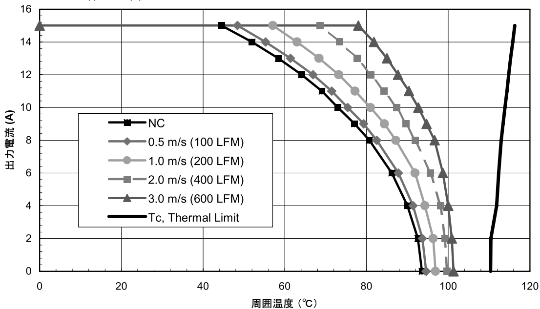
図A-5 iEA48015A050V-001-R 出力電流ディレーティングカーブ
