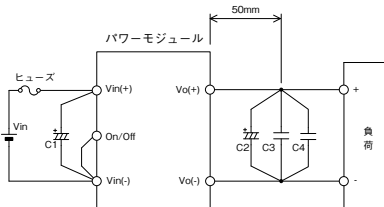
図1-2 基本的な接続
