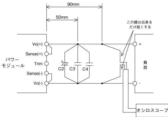
図5-1出力リップル電圧（含スパイクノイズ）測定方法
