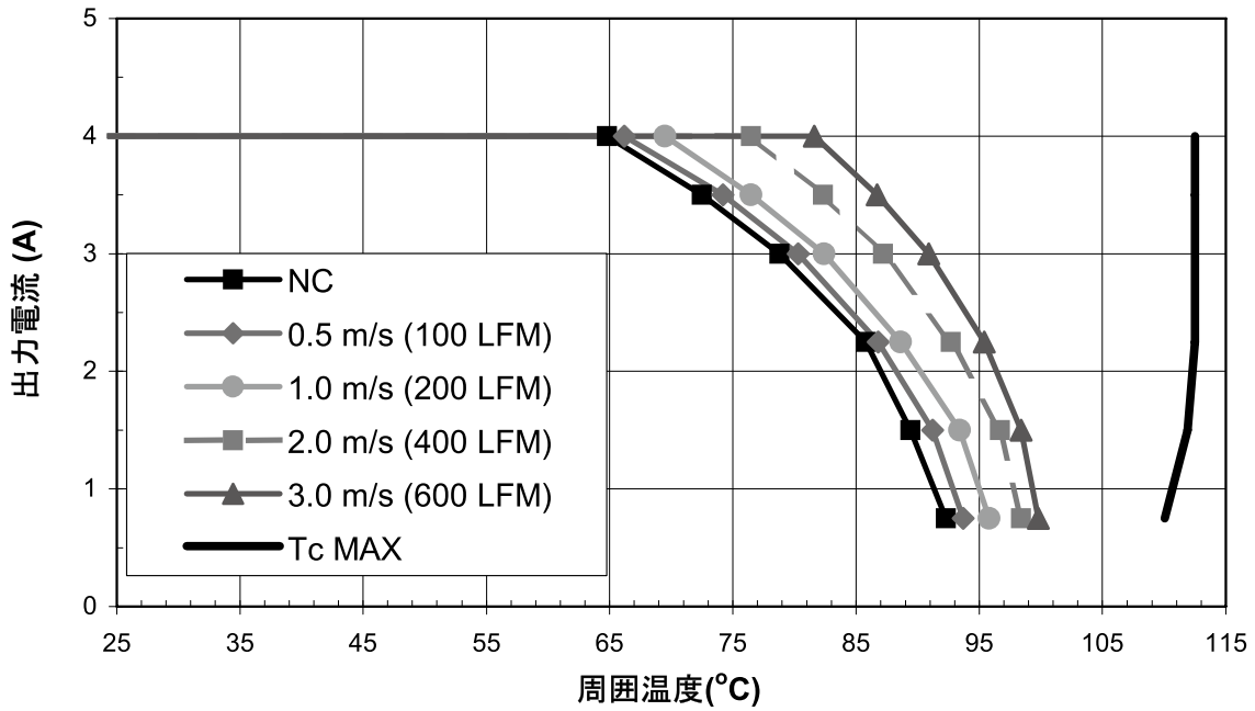
図A-11 iEE4W004A120V-003-R 出力電流ディレーティングカーブ
