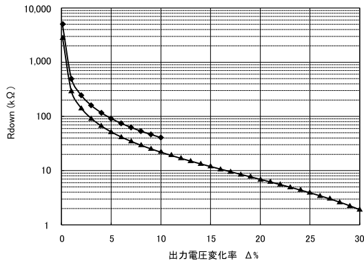
図6-2 △(%)對外付け抵抗
