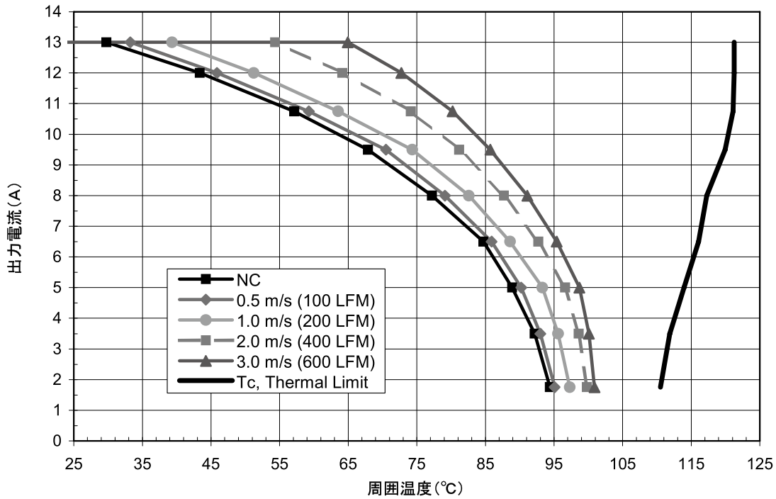
図A-9 iEE48013A050V-003-R 出力電流ディレーティングカーブ
