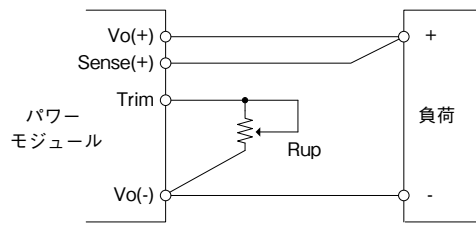
図6-7 可変抵抗接続
