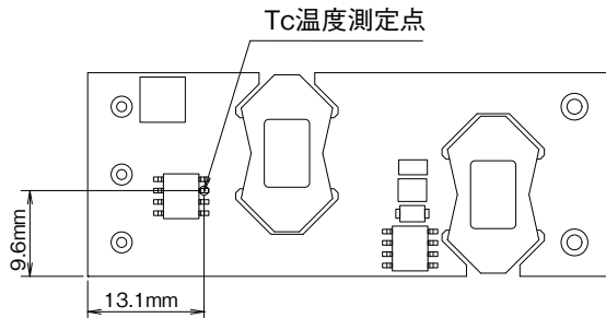
図A-4 パワーモジュール上のTc 測定点
