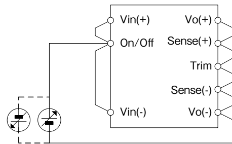
図15-1 入力-出力間電圧試験方法
