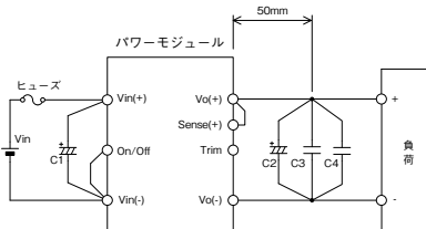
図1-3 基本的な接続
