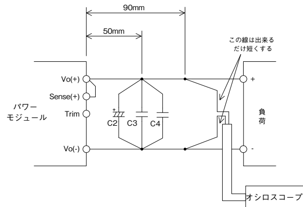
図5-3出力リップル電圧（含スパイクノイズ）測定方法
