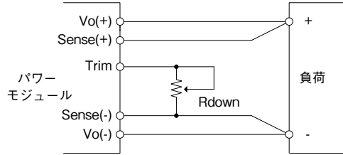
図6-1 可変抵抗接続
