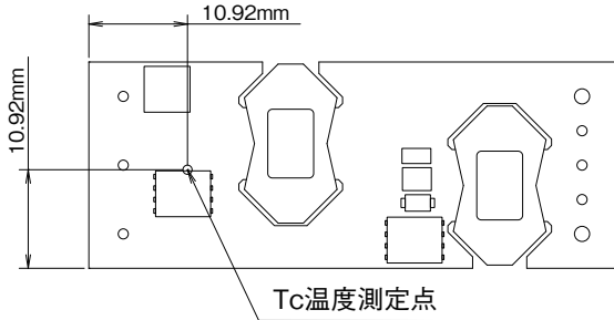
図A-3 パワーモジュール上のTc 測定点
