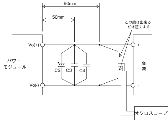
図5-2出力リップル電圧（含スパイクノイズ）測定方法
