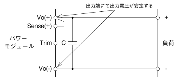
図10-4 リモートセンシングしない場合 (ローカルセンシング)
