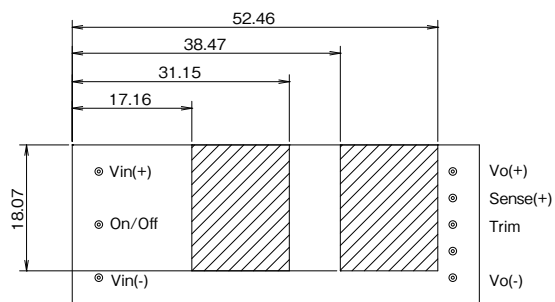
パワーモジュールパターン配線禁止領域(上面透視図)
