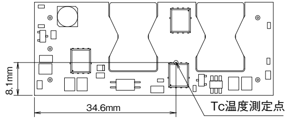
図A-6 パワーモジュール上のTc測定点
