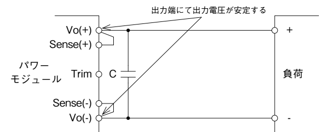
図10-2 リモートセンシングしない場合 (ローカルセンシング)
