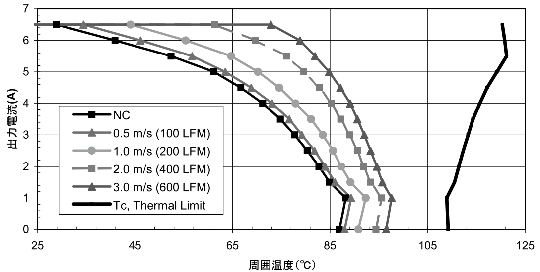
図A-6 iEA48007A120V-001-R 出力電流ディレーティングカーブ
