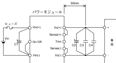
図1-1 基本的な接続
