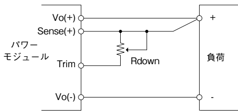
図6-5 可変抵抗接続
