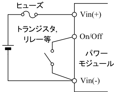
図11-1 On/Off接続例
