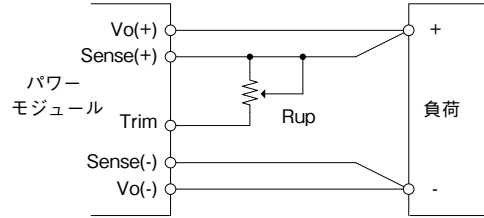
図6-3 可変抵抗接続
