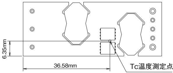
図A-2 パワーモジュール上のTc 測定点
