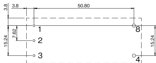
基板穴 (上面視)
