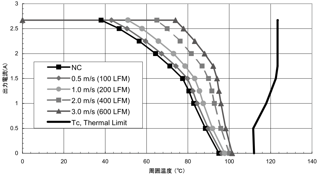
図A-7 iEA48003A280V-001-R 出力電流ディレーティングカーブ
