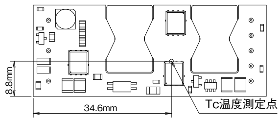
図A-5 パワーモジュール上のTc測定点
