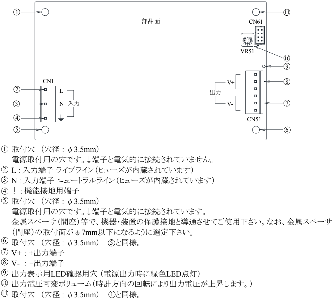
CN61のピン配置と機能
