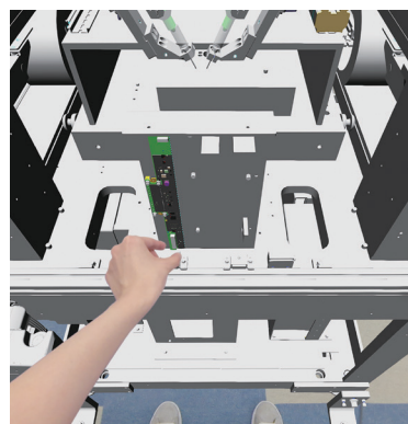
設計CADデータを使用した、作業性検証 自身の手と足元が見えるので、リアルな検証が可能
