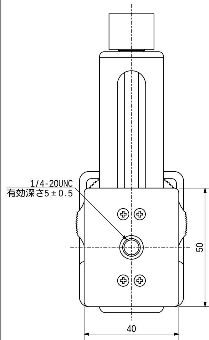
矢視A 背面図
