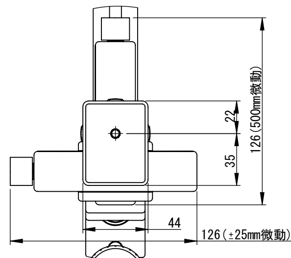
詳細図 A スケール 2 : 5
