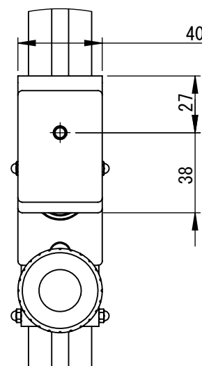
詳細図 A
