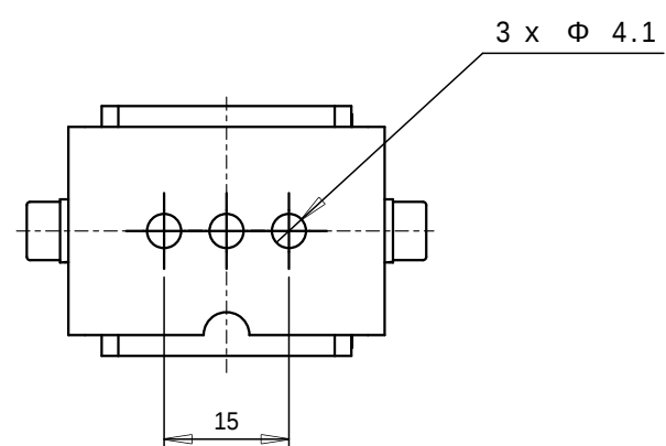
矢視 A スケール 1 : 1
