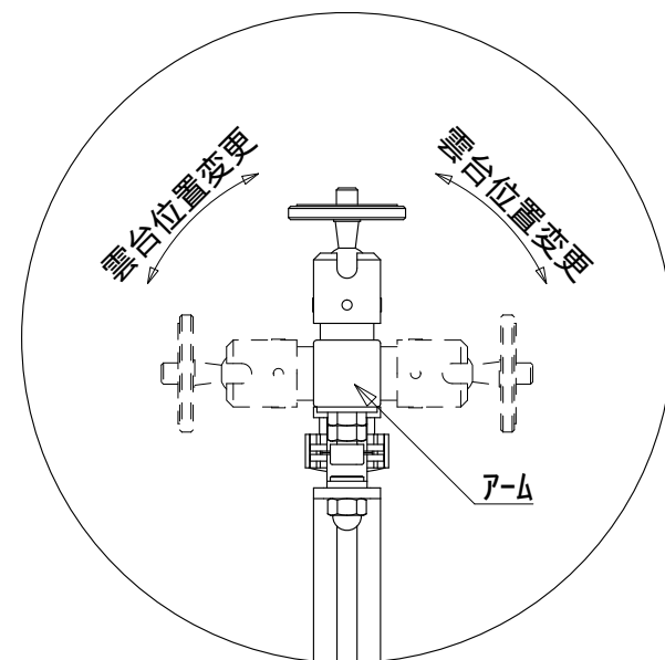
詳細図 A 雲台位置変更 要アーム差替
