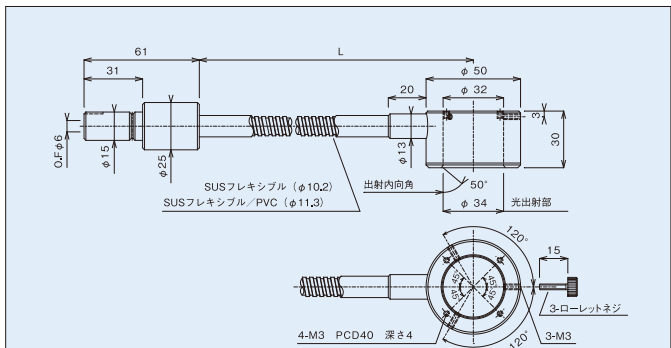
PLG-TR32(L)(P)
