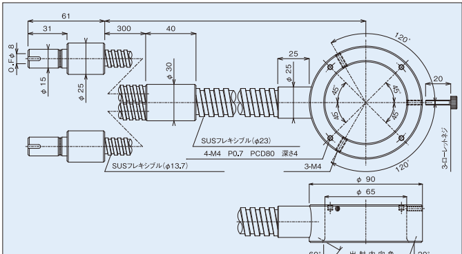
PLG-YDR65(L)
