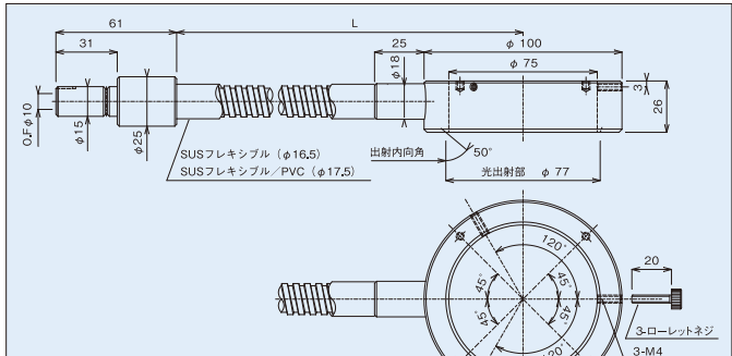
PLG-TR75(L)(P)
