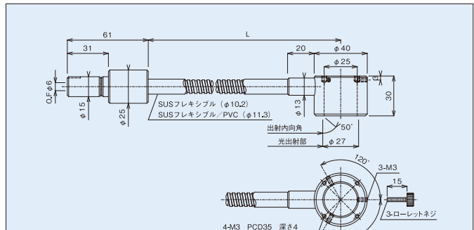
PLG-TR25(L)(P)
