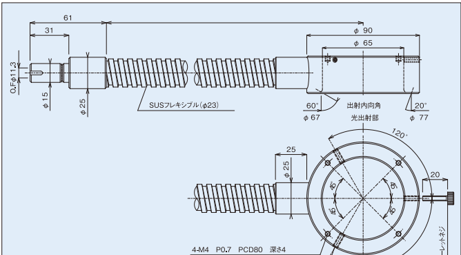
PLG-DR65(L)
