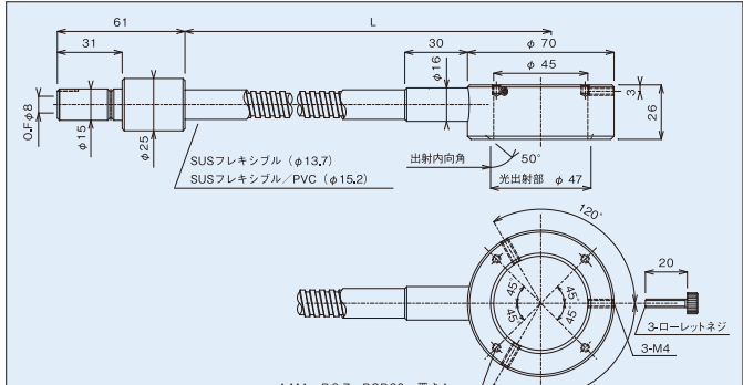
PLG-TR45(L)(P)
