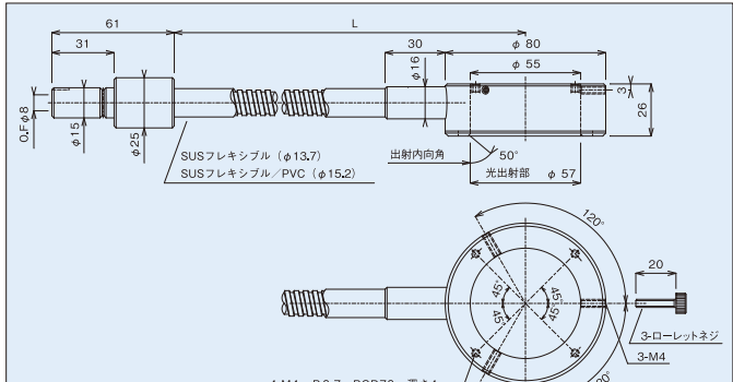
PLG-TR55(L)(P)
