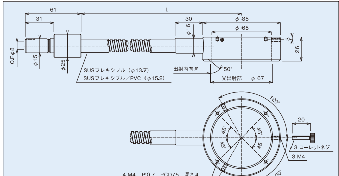
PLG-TR65(L)(P)
