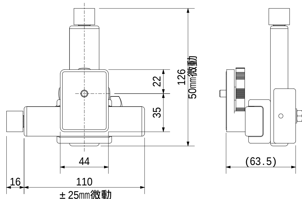
カメラ取付部 詳細
