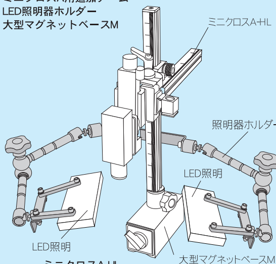
ミニクロスA-HL 照明器ホルダーLED-U(ツイン) 大型マグネットベースM
