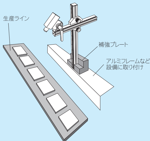
ミニクロス用補強プレート使用例
