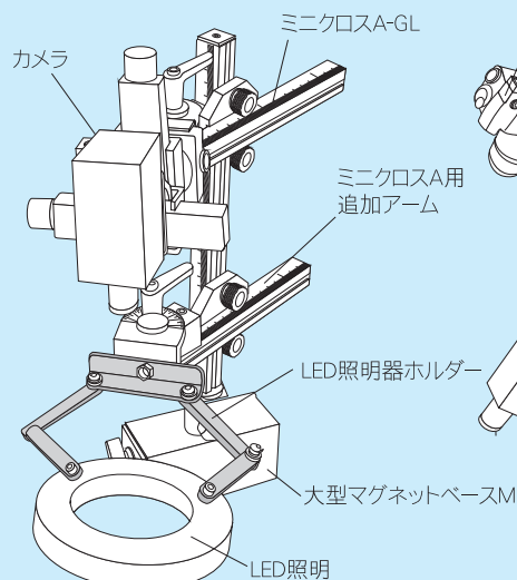
ミニクロスA-GL ミニクロスA用追加アーム LED照明器ホルダー 大型マグネットベースM
