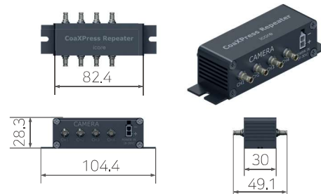
Figure 3 iPLUS-CXPR-DIN4
