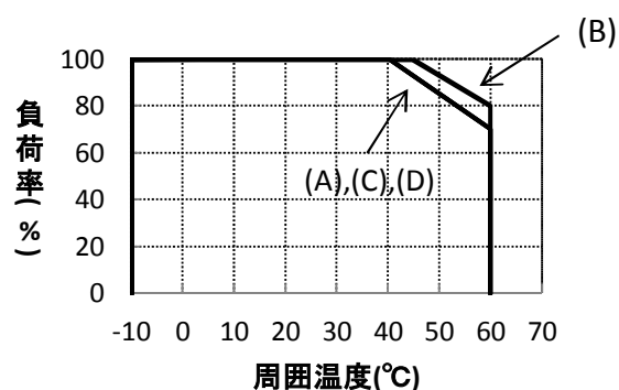
LFS150A-30,48
